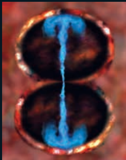
Ampulheta: jatos criam bolhas de gás acima e abaixo do buraco negro
