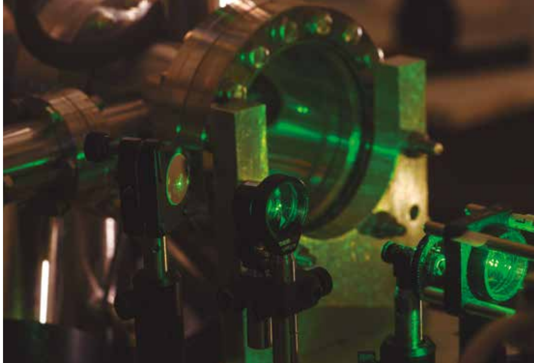
Janela traseira da câmara usada para deixar passar a luz que se deseja coletar
